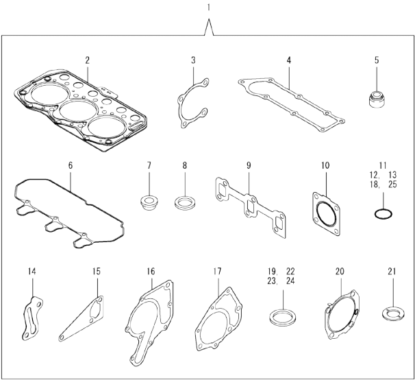
Fig.16. GASKET SET
